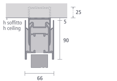
Binario a soffitto Ceiling rail
