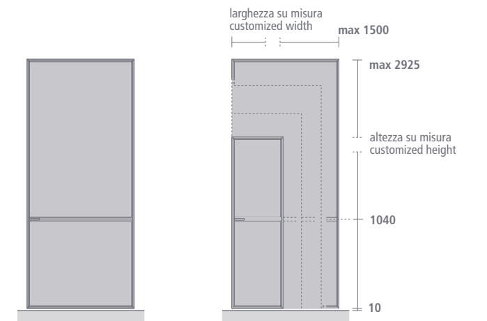
Pannello con traverso Cross panel
